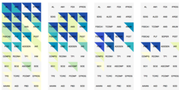
Figura 3. Visualização multi-matricial
